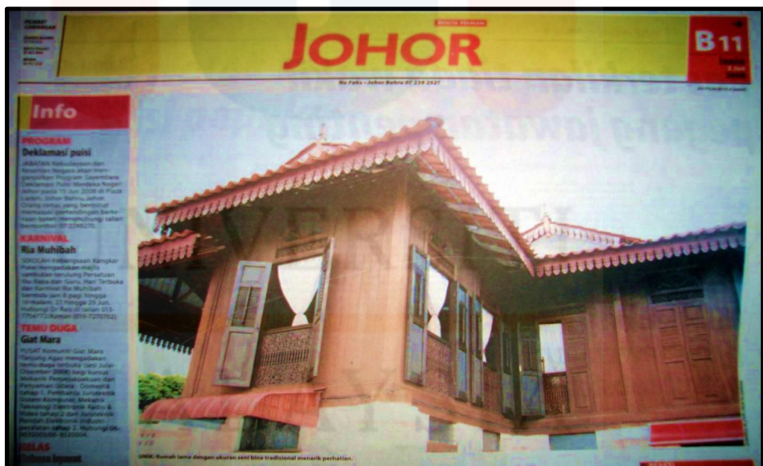
Rajah 2.19: Rumah tradisional Melayu Johor Tuan Zaaba (Sumber: Berita Harian, 3 Jun 2008)
