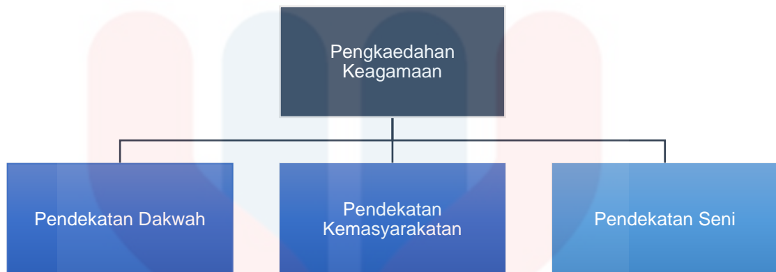
Carta 3.4.2: Jenis Pengkaedahan Keagamaan
